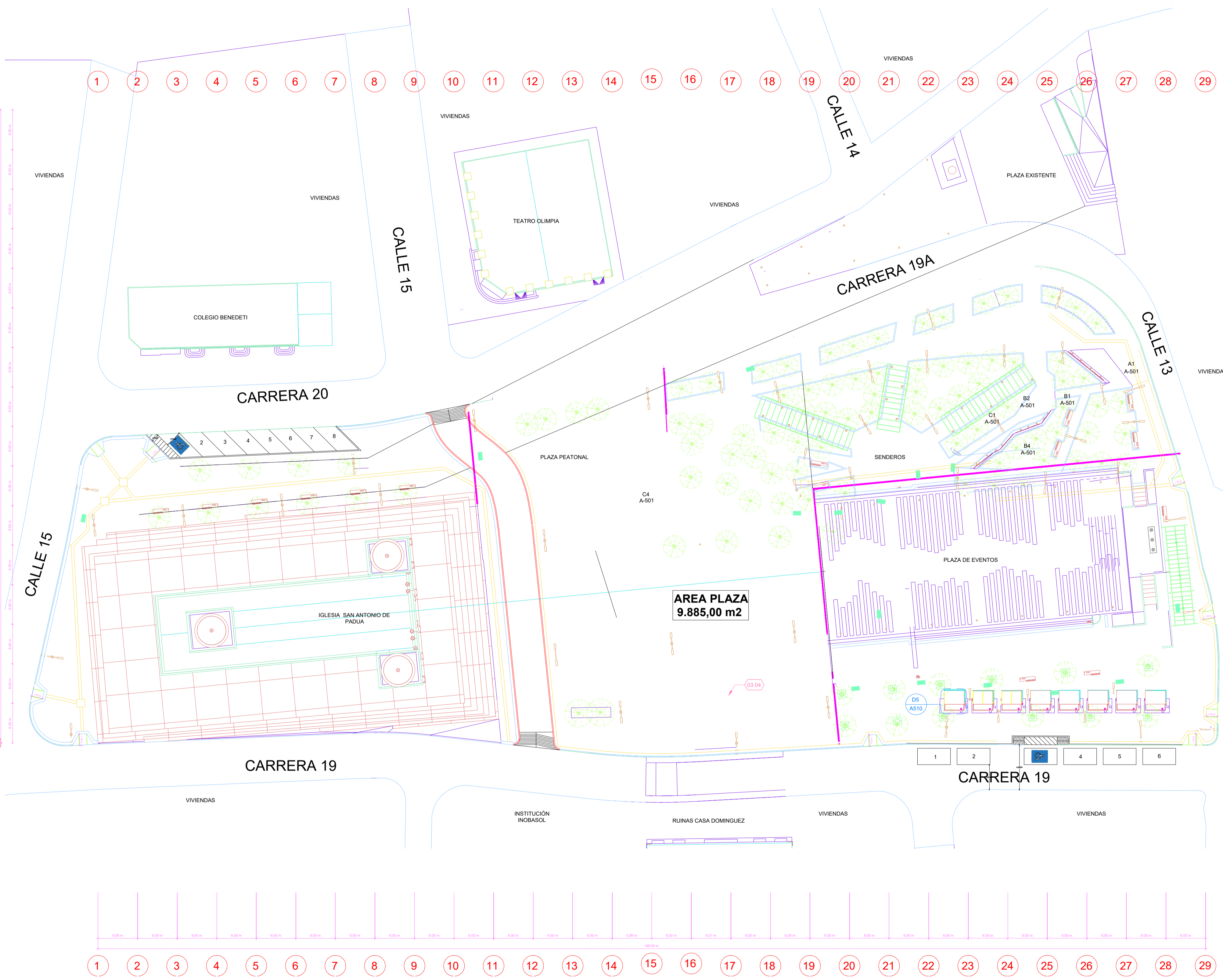
A1 PLANTA GENERAL ESCALA: 1 : 250
